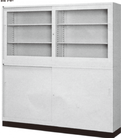
□セット寸法/W1760×D400×H1850mm TG-63SG W1760×D400×H880mm TG-63SS W1760×D400×H880mm T-63B W1760×D380×H90mm
