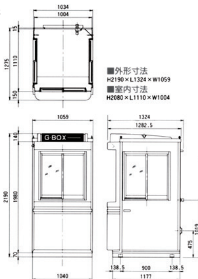
■G-BOX寸法
