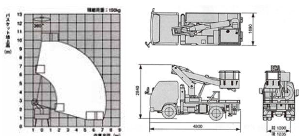
作業範囲図
