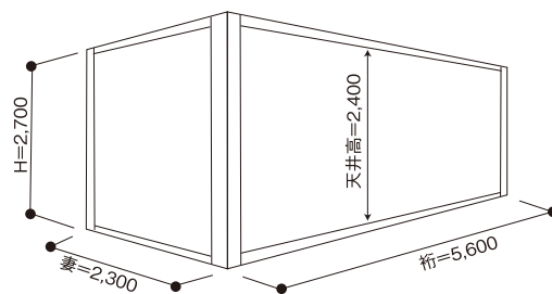
KS-56型 4連棟 2階建て
