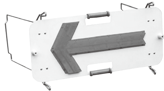
ソーラー式フラッシャーパネル サイズ/H360×W870(mm) 質量/約8kg
