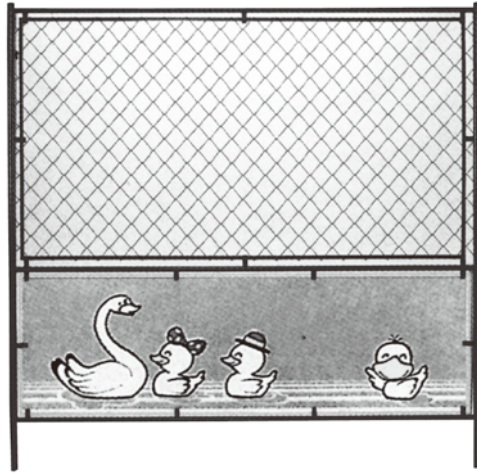
(1017) メッキフェンス1800型 白鳥 サイズ/H1800×W1800(mm) 質量/約16.5kg
