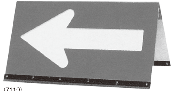
ガルバニウム山形矢印板 サイズ/H450×W900(mm) 質量/約11kg
