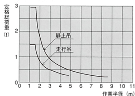
定格総荷重線図
