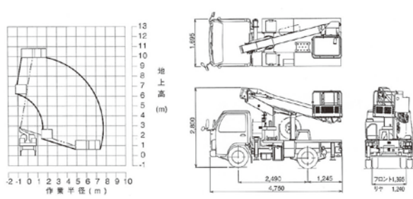
作業範囲図
