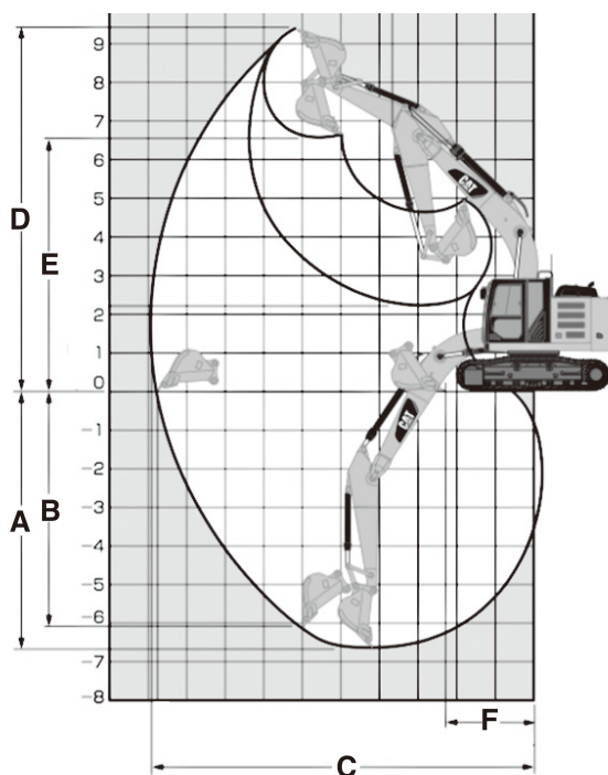
作業範囲
