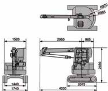
車両寸法図
