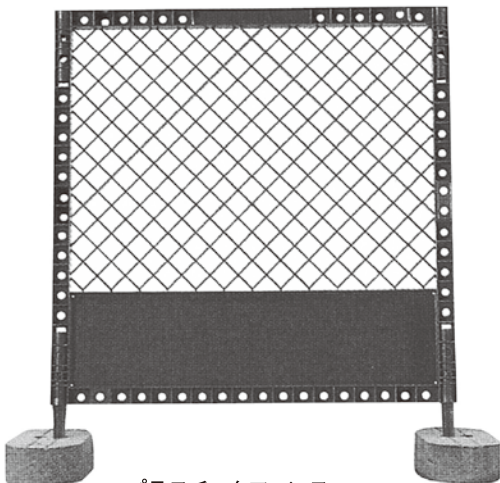
(1112) プラスチックフェンス サイズ/H1100×W1000(mm) 質量/約3.7kg
