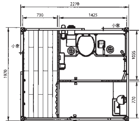
W2270×D1970×H2700/重量約710kg 給水タンク40L/便槽120L
