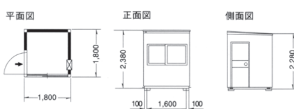
スーパーハウスKs-31型
