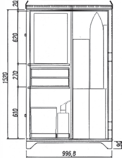
本体内部
