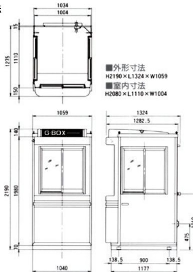
■G-BOX寸法
