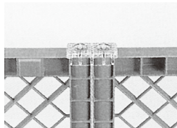
(1116) プラスチックフェンス用 ジョイント
