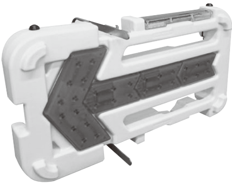
壊れにくい矢印板 サイズ/H464×W779×D105(mm) 質量/約5.8kg
